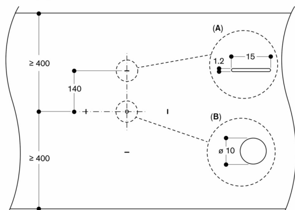
Вид сверху
