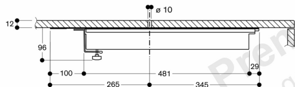
Продольный разрез
