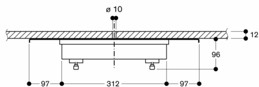
Поперечный разрез
