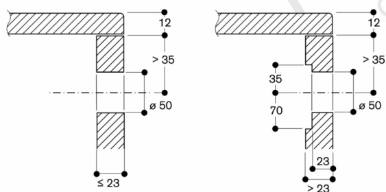
Монтаж ручки управления
